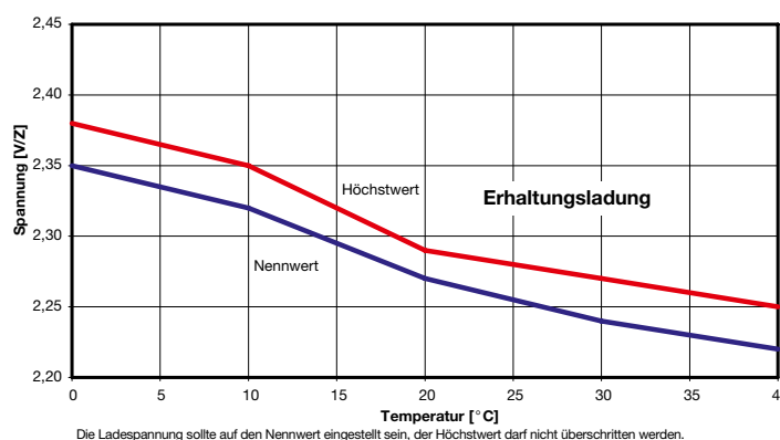
Bild 1: Marathon L/XL und Powerfit S; Ladespannung über der Temperatur
