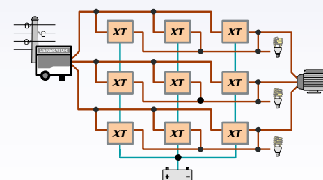
Parallèle + triphasé
