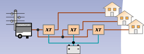
Système centralisé
