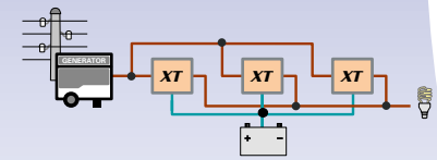
Parallèle
